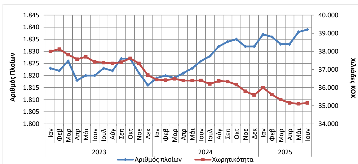
Γράφημα 1: Δύναμη και Ολική Χωρητικότητα των ελληνικών εμπορικών πλοίων 100 ΚΟΧ και άνω, σε μηνιαία βάση, Ιανουάριος 2023 – Ιούνιος 2025
