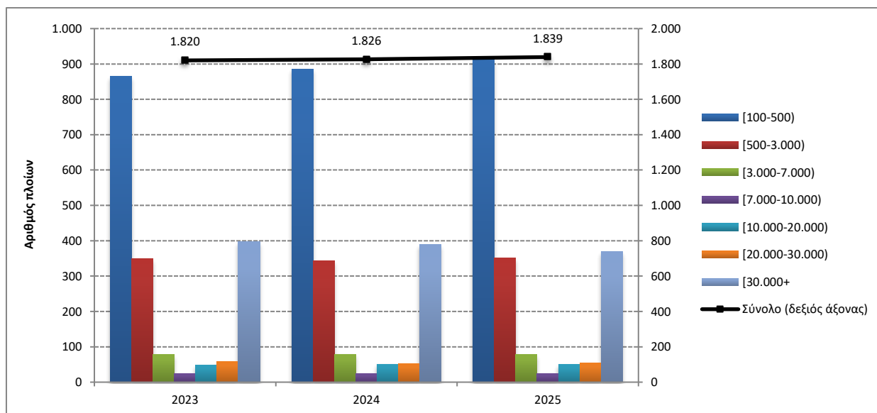
Γράφημα 3: Κατανομή των ελληνικών εμπορικών πλοίων 100 ΚΟΧ και άνω, κατά κλιμάκια ολικής χωρητικότητας, Ιούνιος 2023 – 2025
