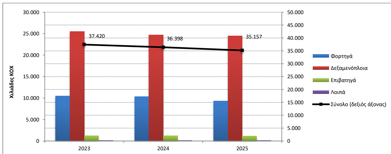
Γράφημα 2β: Χωρητικότητα των ελληνικών εμπορικών πλοίων 100 ΚΟΧ και άνω, κατά κατηγορίες πλοίων, Ιούνιος 2023 – 2025
