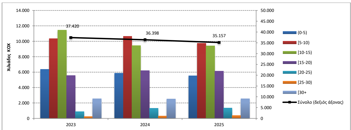
Γράφημα 4β: Κατανομή χωρητικότητας των ελληνικών εμπορικών πλοίων 100 ΚΟΧ και άνω, κατά ομάδες ηλικιών, Ιούνιος 2023 – 2025
